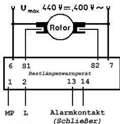
Anschlußschema
